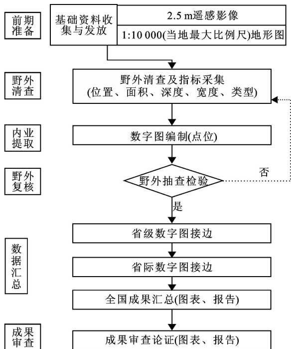
图 3 崩岗普查流程图
