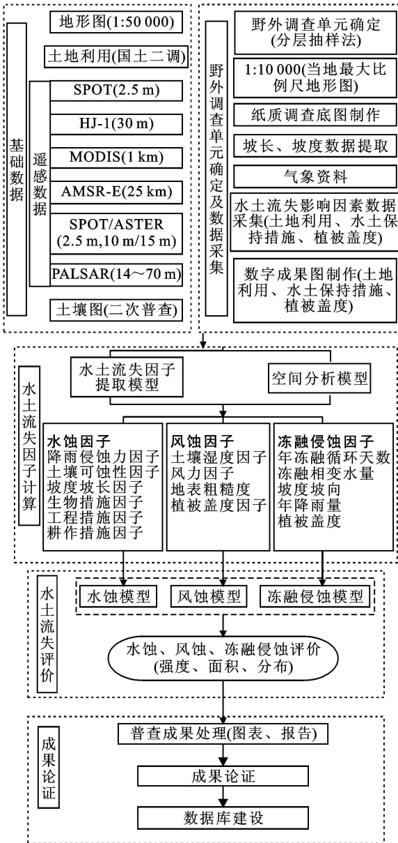
图1 水土流失普查流程图
